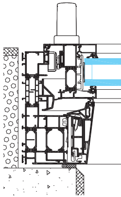
Coupe horizontale - ouvrant caché
