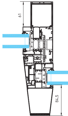
Meneau central - version renforcée
