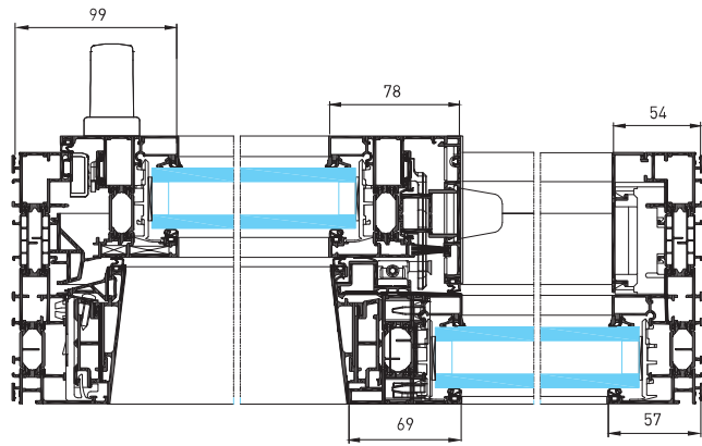
Coupe horizontale - 1 vantail + fixe
