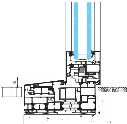
Coupe verticale - partie ouvrant, seuil encastré
